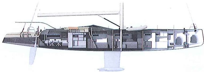
La sezione degli interni del Vismara V80: si notano l'ampio quadrato posizionato a poppa e l'accesso sottocoperta, attraverso una scala, direttamente dal pozzetto rialzato.
